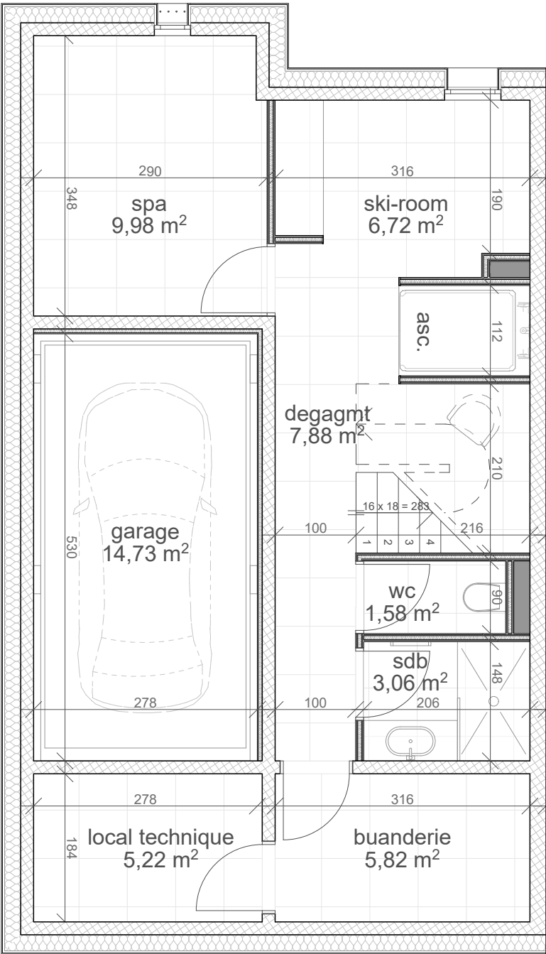
Niveau sous-sol
