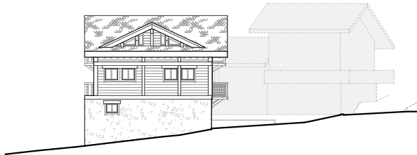
Façade Sud-Ouest
