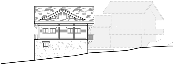
Façade Sud-Ouest
