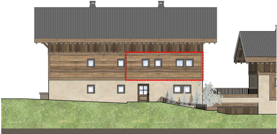
FACADE NORD
