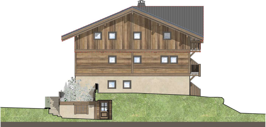
FACADE OUEST
